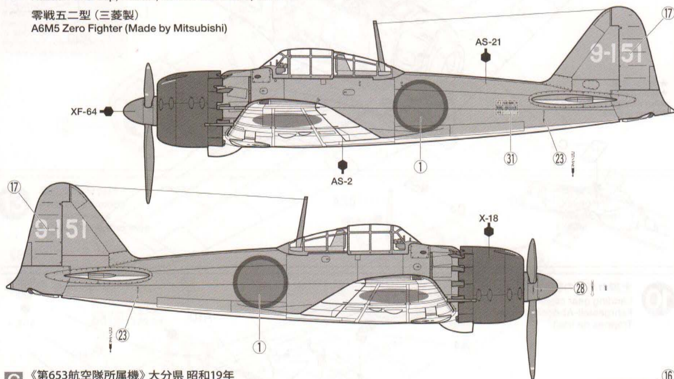
C 《第653航空隊所属機》 大分県 昭和19年 653rd Air Group, Oita Prefecture, 1944 零戦五二型 (中島製) A6M5 Zero Fighter (Made by Nakajima)
